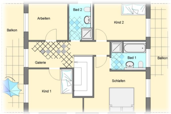
Grundriss Dachgeschoss
