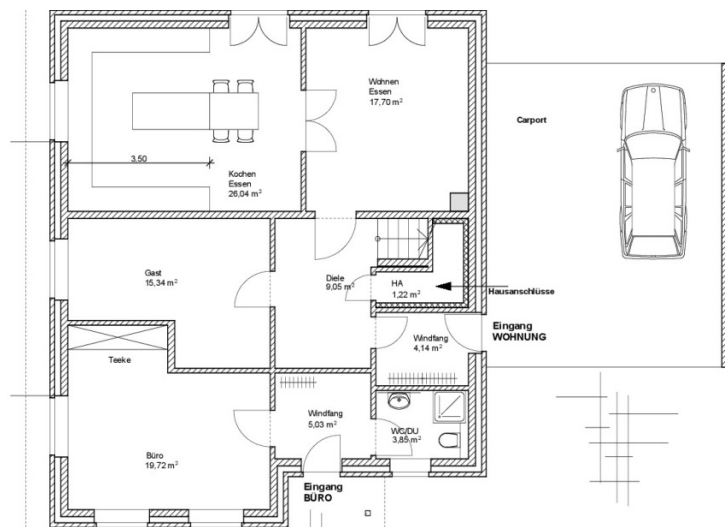
Grundriss Erdgeschoss
