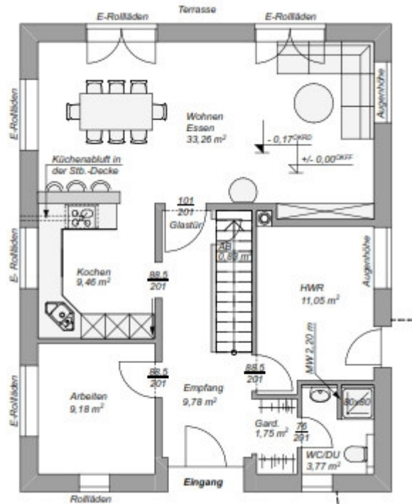
Grundriss Erdgeschoss
