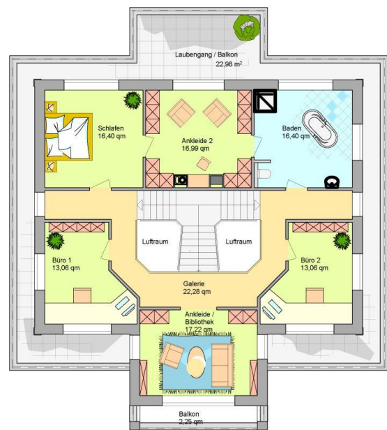
Grundriss Dachgeschoss
