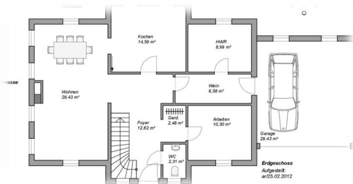
Grundriss Erdgeschoss
