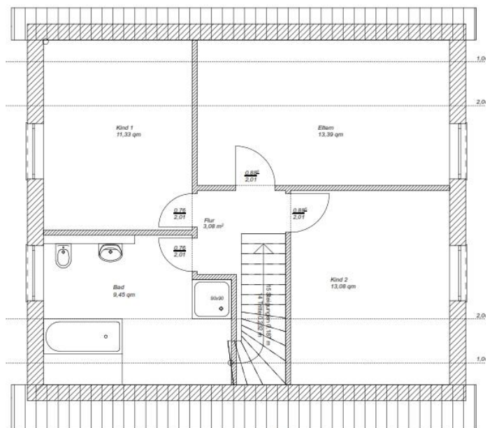
Grundriss Dachgeschoss
