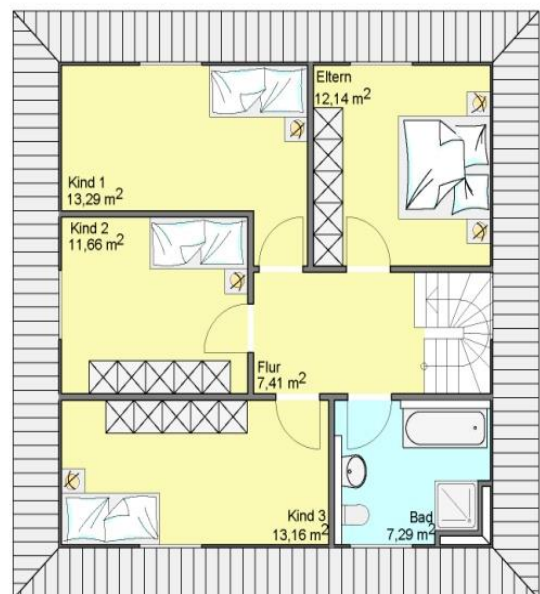
Grundriss Dachgeschoss
