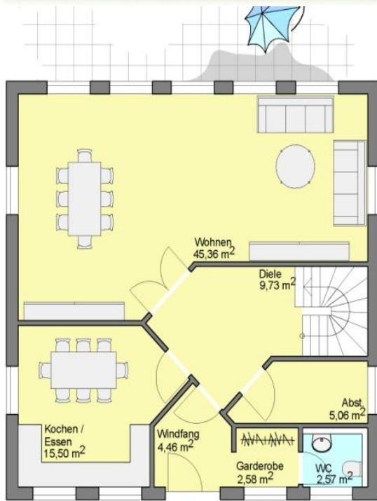
Grundriss Erdgeschoss
